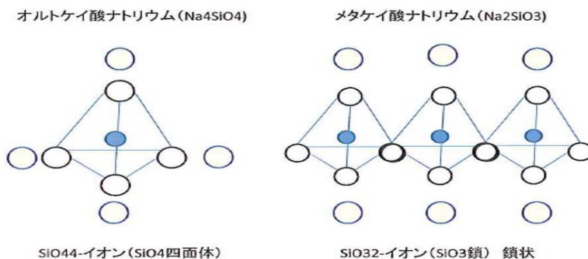
図1 ケイ酸塩イオンの構造
